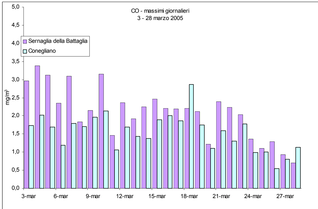
Figura 2 –Valori massimi di monossido di carbonio CO rilevati presso la stazione fissa di Conegliano e il Laboratorio Mobile posizionato a Sernaglia della aBattaglia
