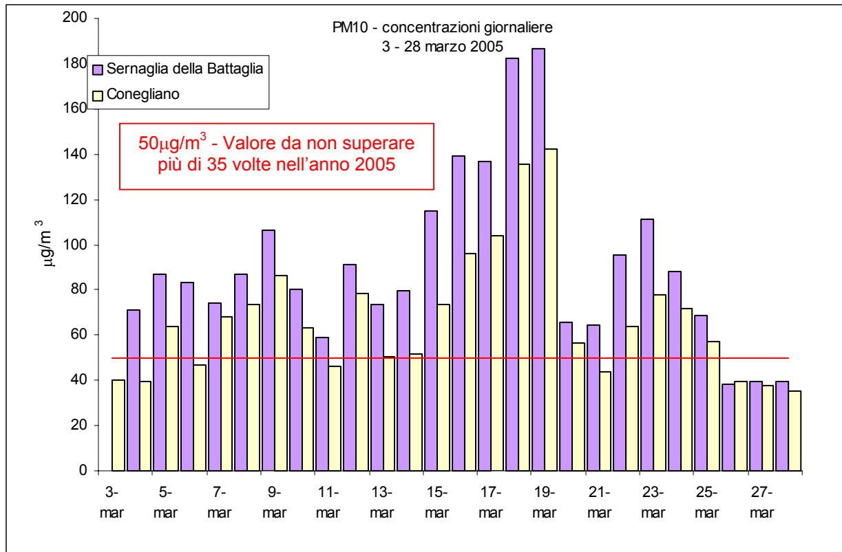
Figura 6 –Valori massimi di polveri inalabili PM10 rilevati presso la stazione di Conegliano e il Laboratorio Mobile posizionato a Sernaglia della Battaglia
