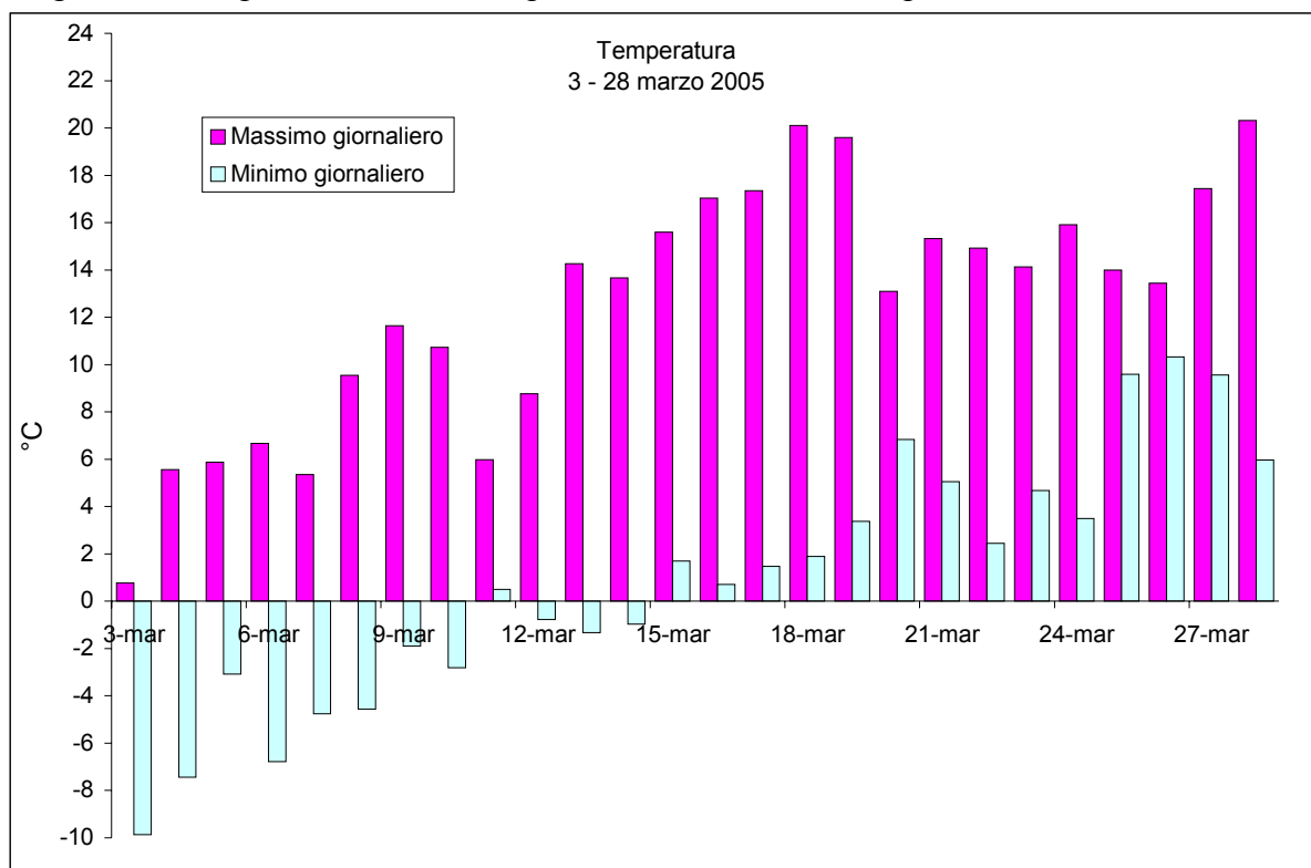
Figura 9 – Valori minimi e massimi di Temperatura rilevati presso il Laboratorio Mobile.
