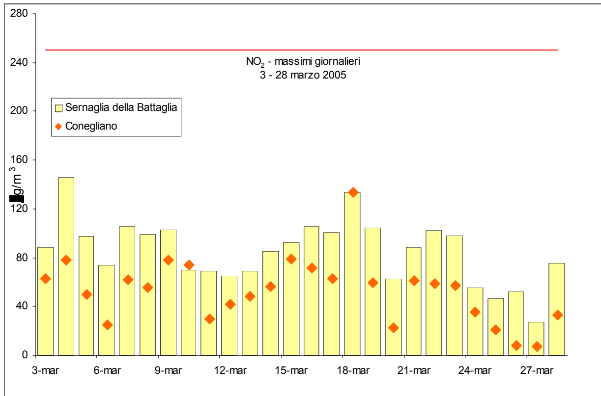
Figura 3 –Valori massimi di biossido di azoto \text{NO}_2 rilevati presso la stazione fissa di Conegliano e il Laboratorio Mobile posizionato a Sernaglia della Battaglia
