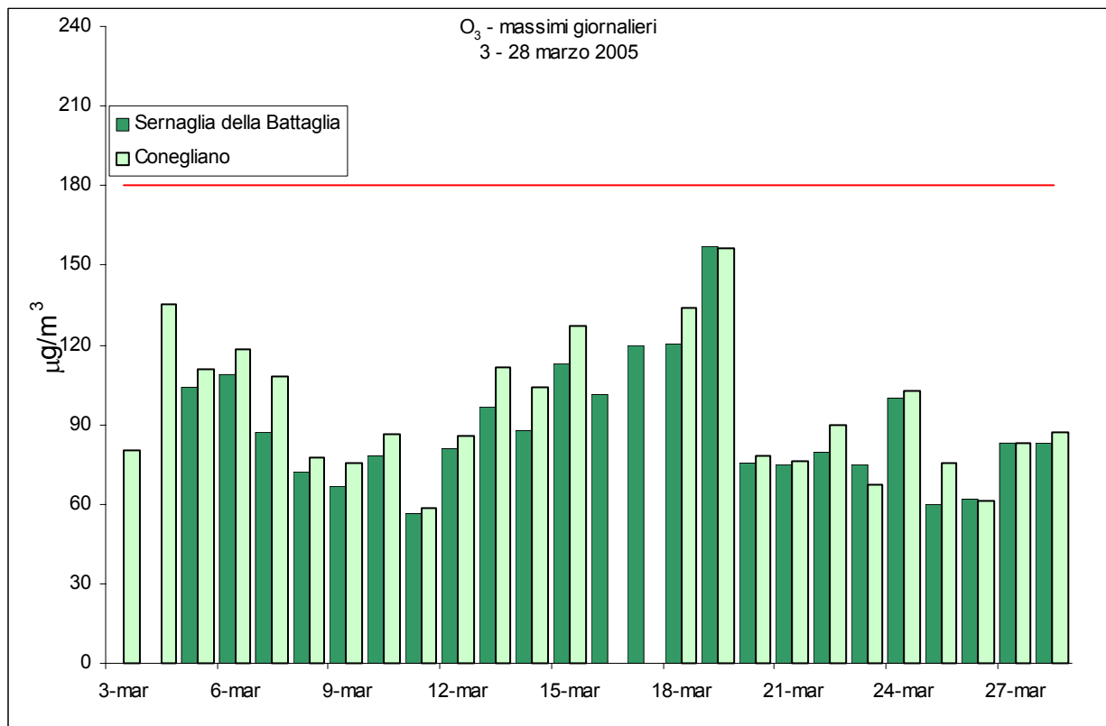
Figura 4 –Valori giornalieri massimi di ozono O 3 rilevati presso la stazione fissa di Conegliano e il Laboratorio Mobile posizionato a Sernaglia della Battaglia
