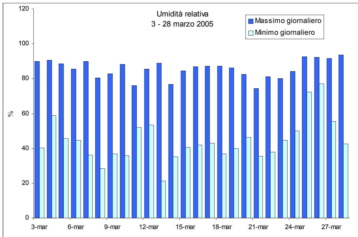
Figura 10 – Valori medi giornalieri di umidità % relativa rilevata presso il Laboratorio Mobile.
