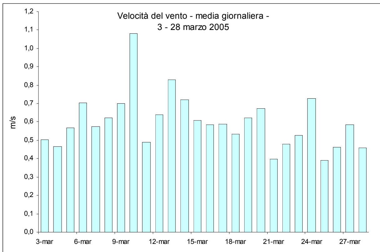
Figura 8 – Valori medi giornalieri della velocità del vento rilevati presso la stazione di Conegliano.
