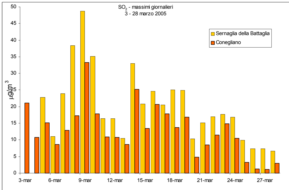
Figura 5 –Valori massimi di biossido di zolfo SO 2 rilevati presso la stazione fissa di Conegliano e il Laboratorio Mobile posizionato a Sernaglia della Battaglia
